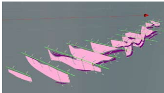
Preliminära sektioner över Fetsjön.
