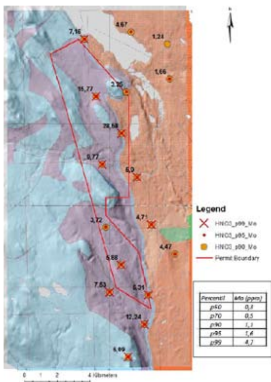
Surberget. Anomalikarta för molybden.
