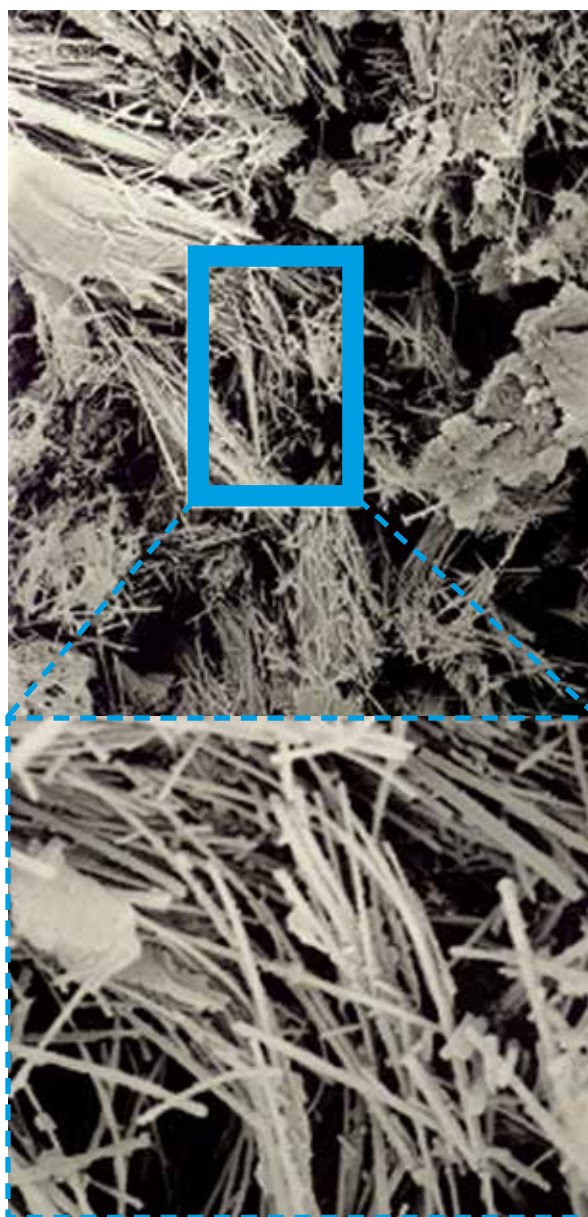
Filtermaterialet Aqualite™ i kraftig förstoring. Bland annat den stora specifika ytan gör Aqualite™ mycket effektiv.
